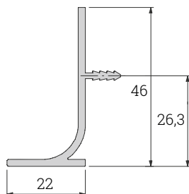
Listwa korytkowa podwójna pionowa C
