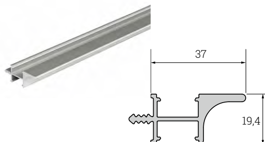
Profil do krawędzi korpusu z dwustronnym LED
