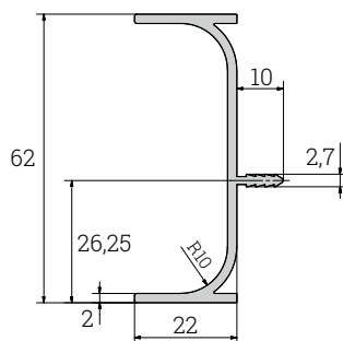
Listwa korytkowa podwójna pionowa C
