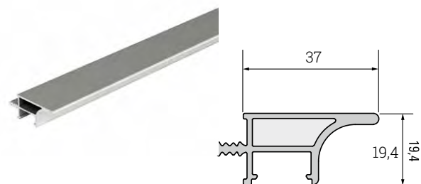
Profil do krawędzi korpusu z jednostronnym LED
